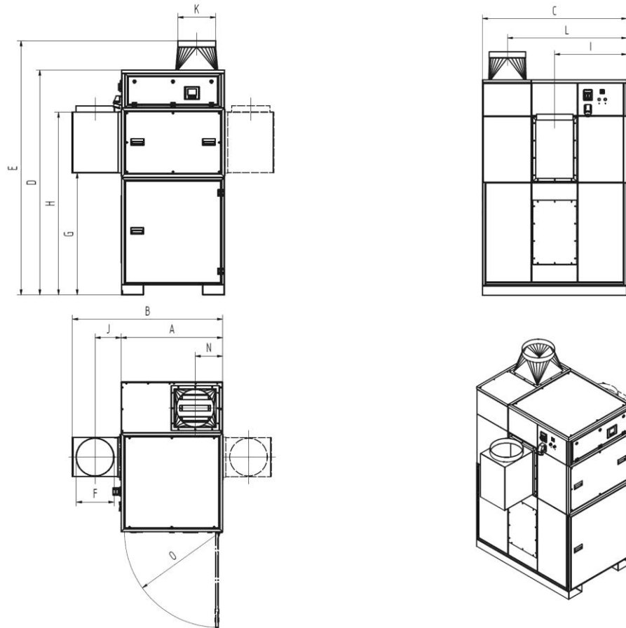
Fig. 59: Dimension sheet 3530
