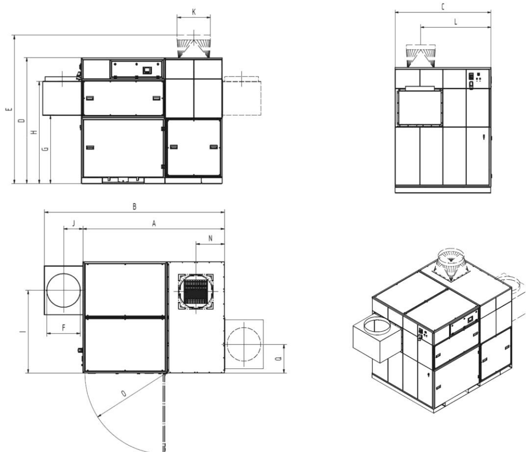
Fig. 65: Dimension sheet 3585
